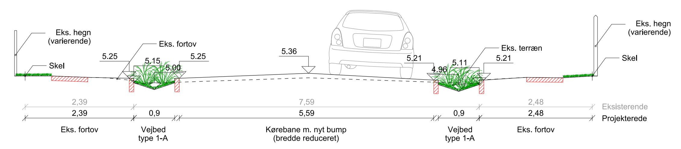
SNIT A 1:50
